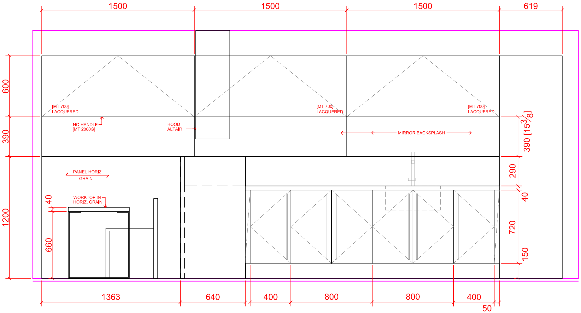
ELEVATION A
