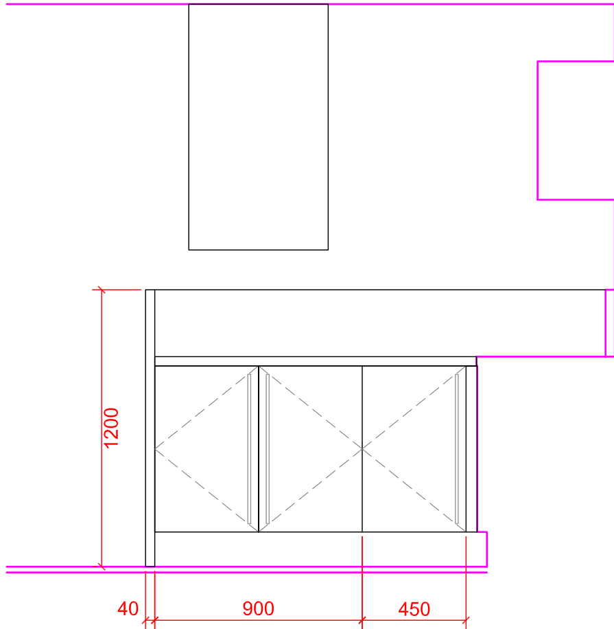
ELEVATION B
